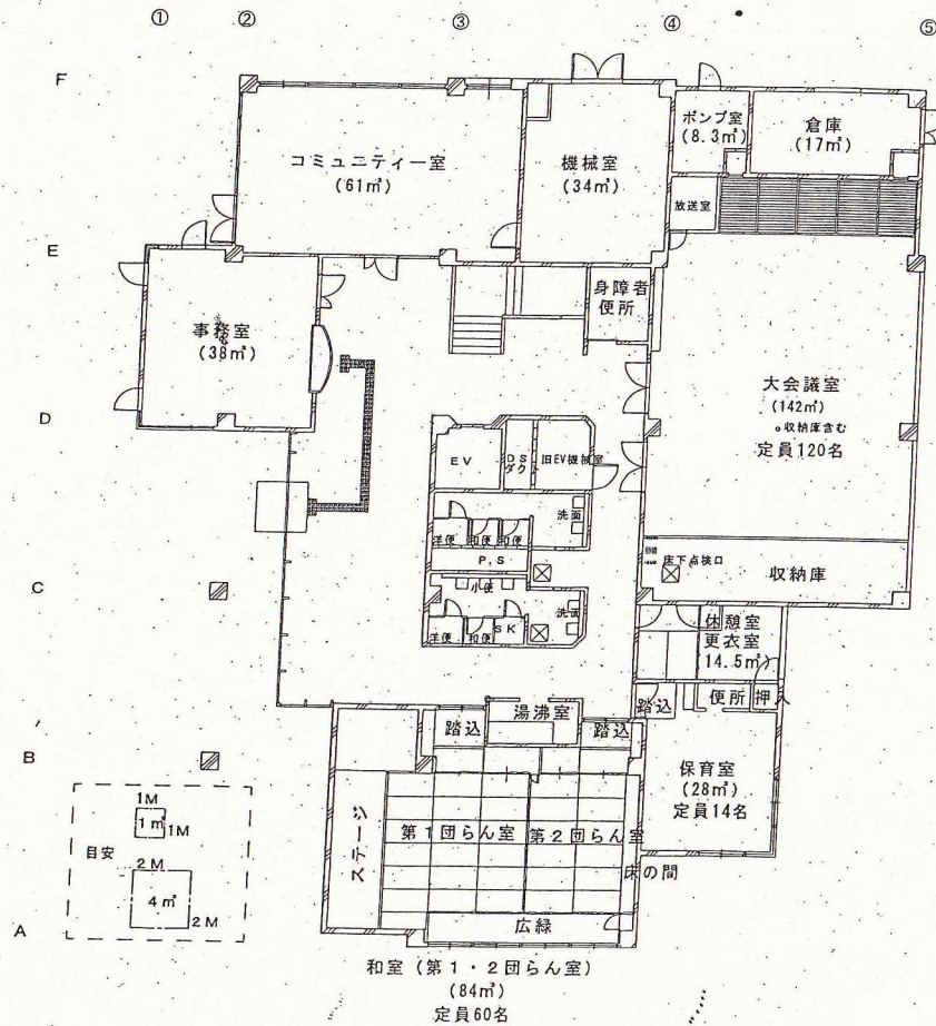
現況図 1階
