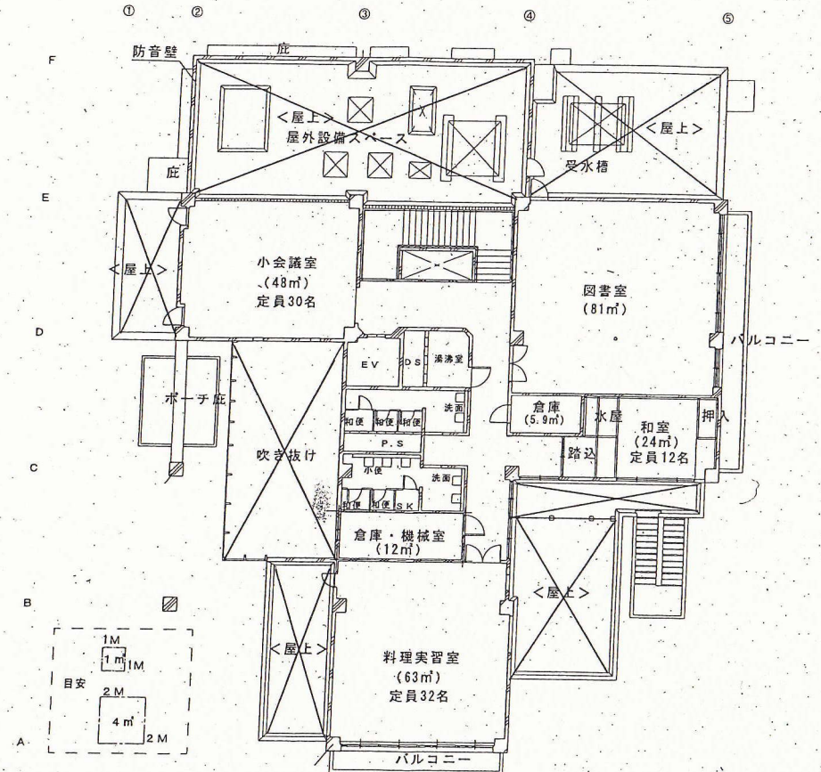
現況図 2階
